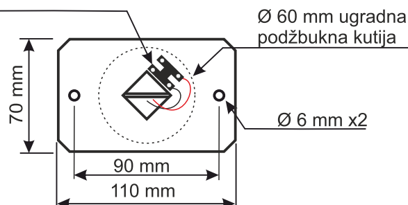
Detalj montaže
