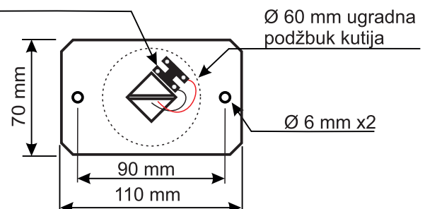
Detalj montaže
